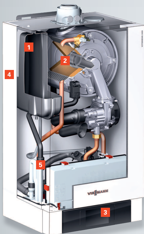
Vitodens 200-W (solotoestel)
